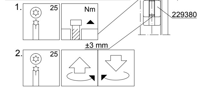
Rollenband für Anschlagtüren
