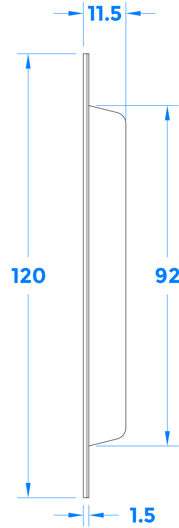
Section A-A
