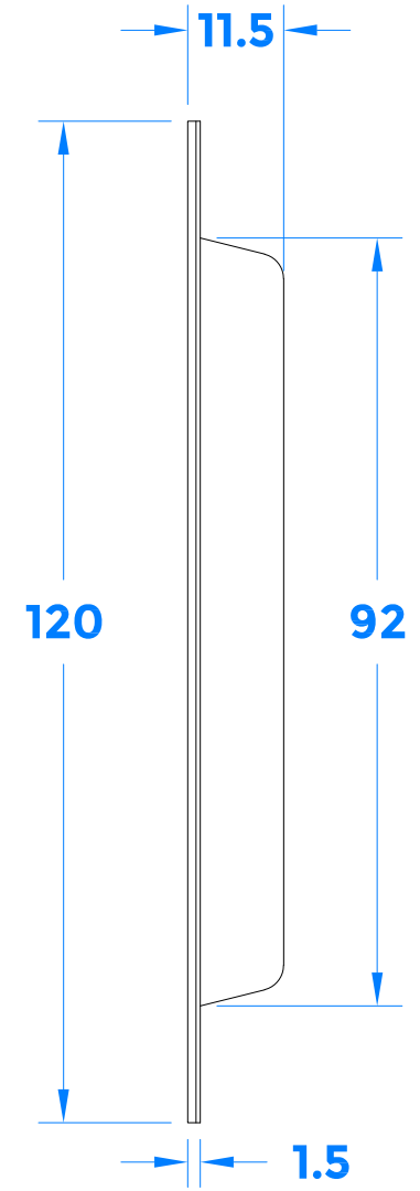
Section A-A
